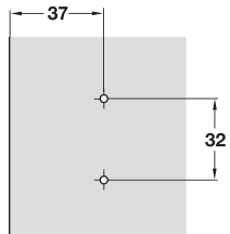
Patrón de perforación
