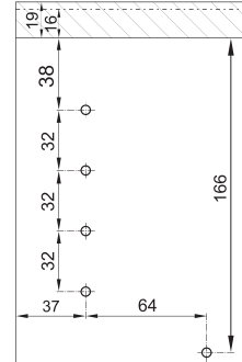
Esquema de taladro costado
