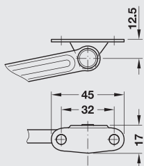
Placa angular para fijar en puertas elevables de madera
