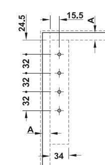
Esquema de taladro de puerta A= Espesor costado-Holguera
