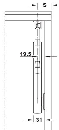
Diagrama de instalación bracket puerta
