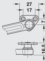
Soporte atornillable para fijar al marco de aluminio
